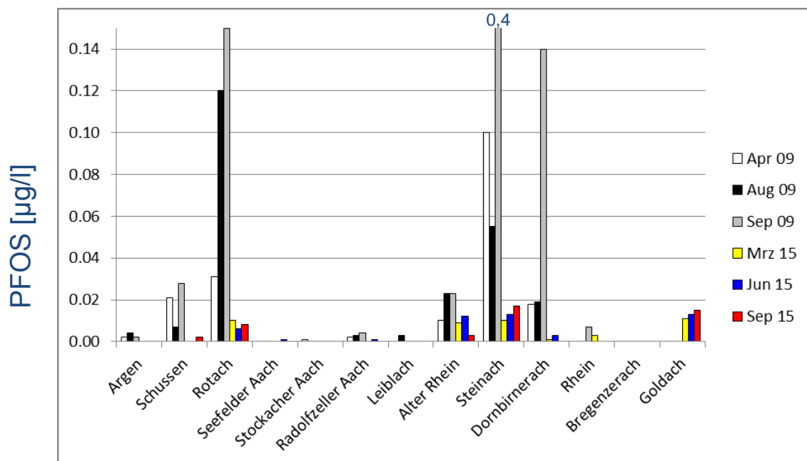
Abbildung 5: Konzentrationen von Perfluorooctansulfonat (PFOS) 2009 und 2015
